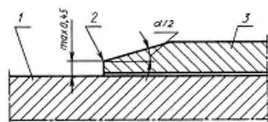
1 — поверхность стебля; 2 — измерительная кромка; 3 — барабан
