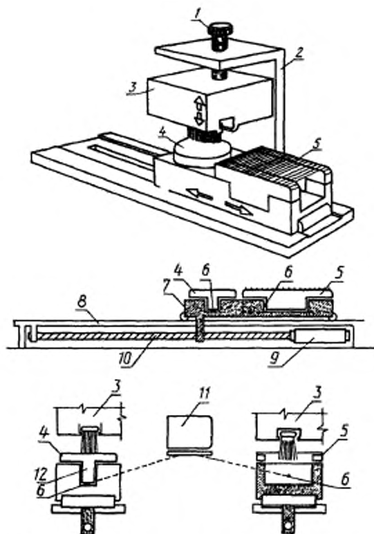
Схема оборудования, применяемого для измерения жесткости
