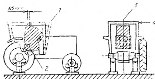
1 — деформация под действием продольного нагружения сиденья; 2 — контрольная точка сиденья; 3 — продольная центральная линия, проходящая через контрольную точку сиденья; 4 — нагрузка
