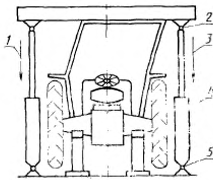
Пример приспособления для приложения вертикальной статической нагрузки
