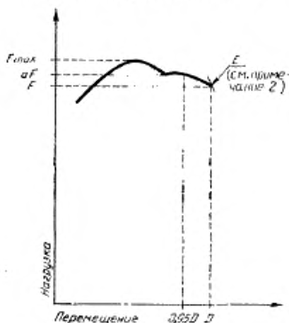
Диаграмма нагрузка — перемещение
