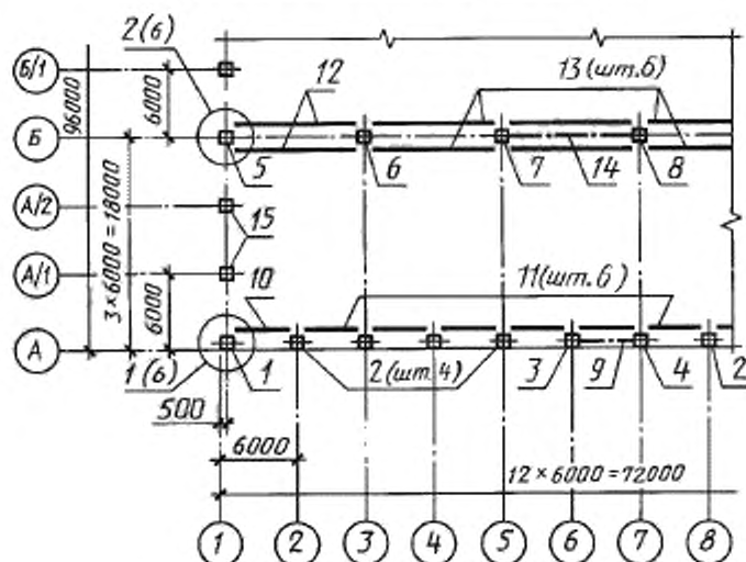
Схема расположения колонн и подкрановых балок
