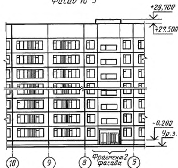
Фасад 10-5
