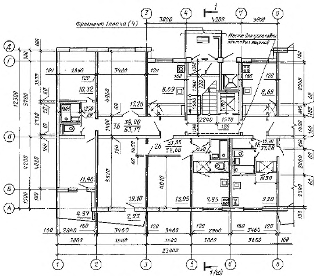
Пример выполнения плана этажа жилого дома
