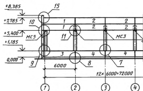
Схема расположения панелей стен
