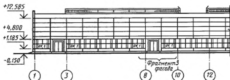
Фрагмент 3 фасада
