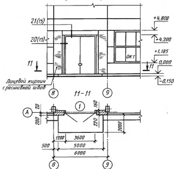
Фрагмент 3 фасада
