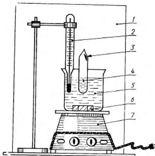
1—защитный экран; 2—термометр; 3—забывшая ампула; 4—исследуемый раствор; 5—теплопроводящая жидкость; 6—мешалка; 7—нагревательный прибор
