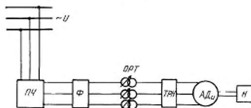
ПЧ — преобразователь частоты (статический или тиристорный); Ф — фильтр; ОРТ — однофазные регулировочные трансформаторы; ТРН — тиристорный регулятор напряжения с фазным управлением; АД u — испытуемый асинхронный двигатель; Н — нагрузка на валу асинхронного двигателя
