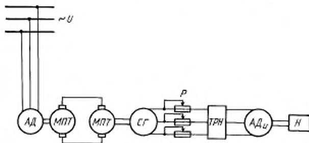
АД — асинхронный двигатель; МПТ — машины постоянного тока; СГ — синхронный генератор; АД—МПТ—СГ — система генератор—двигатель; R — резистор; ТРН — тиристорный регулятор напряжения с фазным регулированием; АД u — испытуемый асинхронный двигатель; Н — нагрузка на валу асинхронного двигателя
