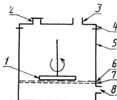
1—магнитная мешалка; 2—предохранительный клапан; 3—патрубок подачи давления; 4—крышка; 5—корпус; 6—испытываемый образец мембраны; 7—дренаж; 8—отверстие для выпуска фильтрата
