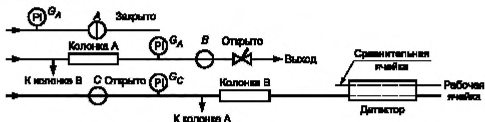
Рисунок 1 — Обратная продувка с изменением давления
