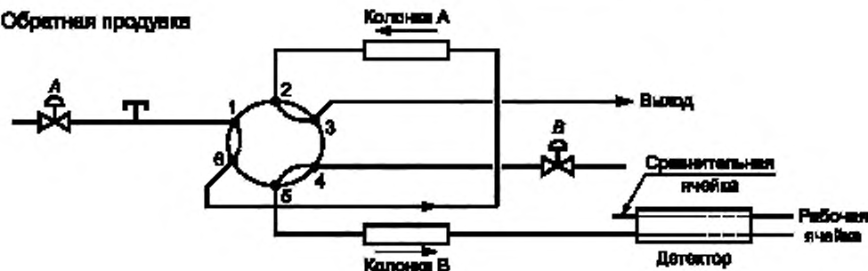
Рисунок 2 — Обратная продувка с переключением клапанов
