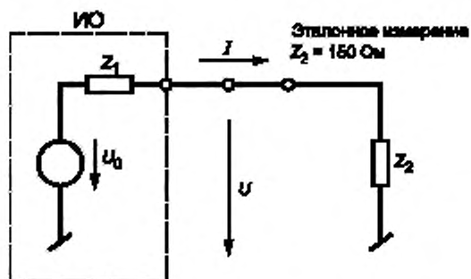
ИО — испытываемое оборудование; Z_1 — общее несимметричное полное сопротивление ИО; U_0 — напряжение источника ИРП; U — общее несимметричное напряжение ИРП на порте связи; I — общий несимметричный ток ИРП на порте связи; Z_2 — общее несимметричное полное сопротивление нагрузки
