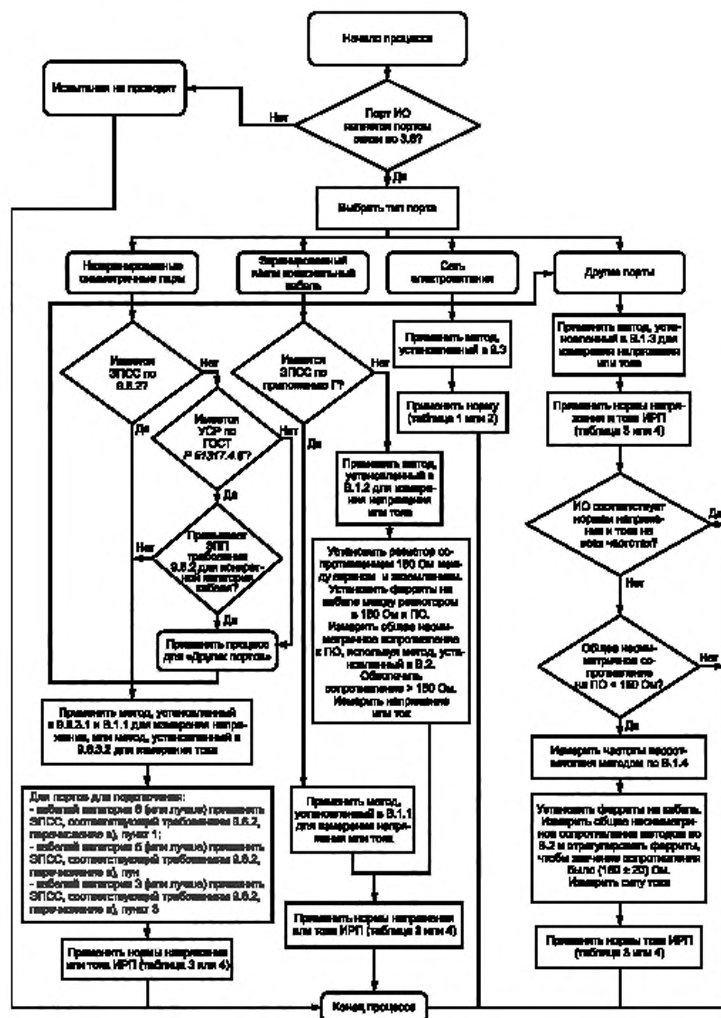
Рисунок В.6 — Алгоритм выбора методов испытаний
