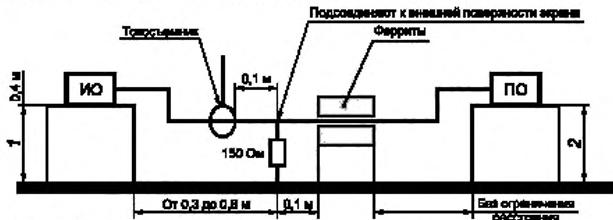
Рисунок В.2 — Применение нагрузки сопротивлением 150 Ом, подключенной к внешней поверхности экранированного кабеля
