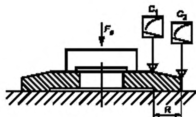
Рисунок В.3 — Испытательное оборудование
