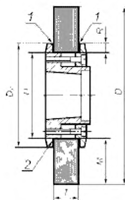
1 — мягкие прокладки; 2 — выточка
