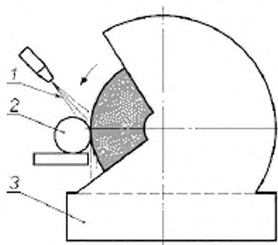
1 — СОЖ; 2 — обрабатываемая деталь, 3 — контейнер для сбора шлама
