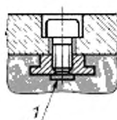
Рисунок В.6 — Правильное расположение гайки и болта
