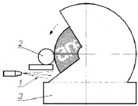
1 — СОЖ; 2 — обрабатываемая деталь; 3 — контейнер для сбора шлама
