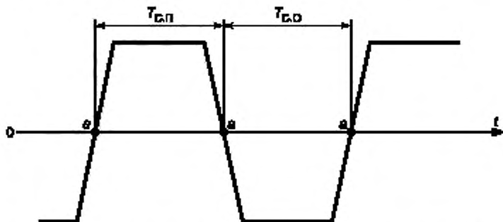
T_{\text{с.п.}} — длительность положительной полу волны сигнала; T_{\text{с.о.}} — длительность отрицательной полу волны сигнала; а — точка перехода сигнала через нулевой уровень (нуль-переход)
