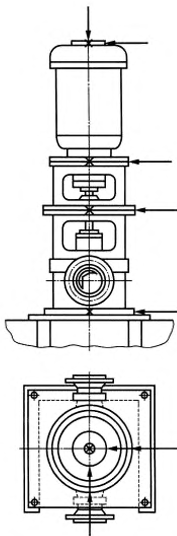
Рисунок 2 — Точки измерений для вертикально установленной машины
