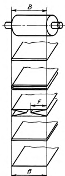
Схема сматывания основных видов пленки в рулон
