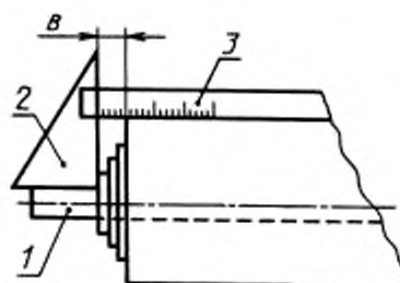
1 — шпуля; 2 — угольник; 3 — линейка
