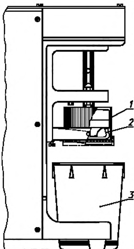
1 — смесительная (промывочная) камера; 2 — тестомесилка; 3 — резервуар для сбора выходящего вещества
