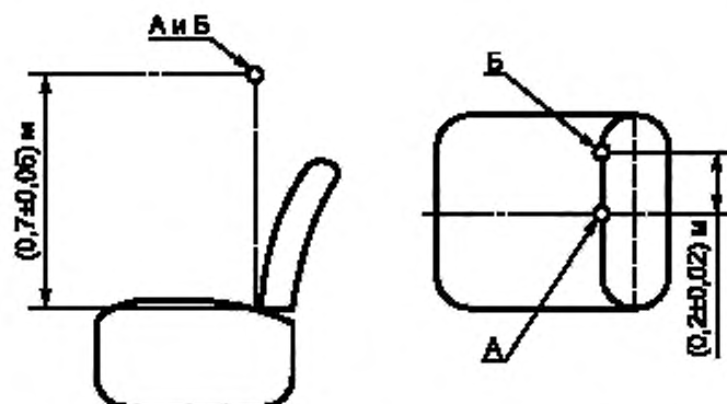
Рисунок 1 — Положение микрофона относительно сиденья
