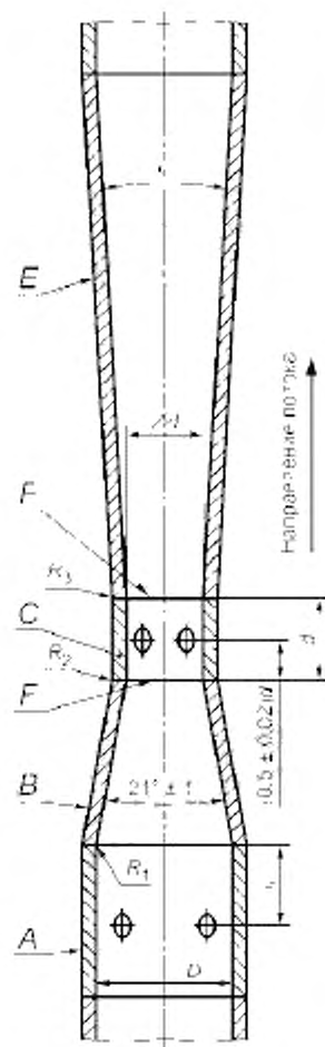
Е — диффузор; С — горловина; В — сужающаяся коническая часть; А — входной цилиндрический участок; F — плоскости соединения элементов трубы Вентури; с — см. 5.4.7
