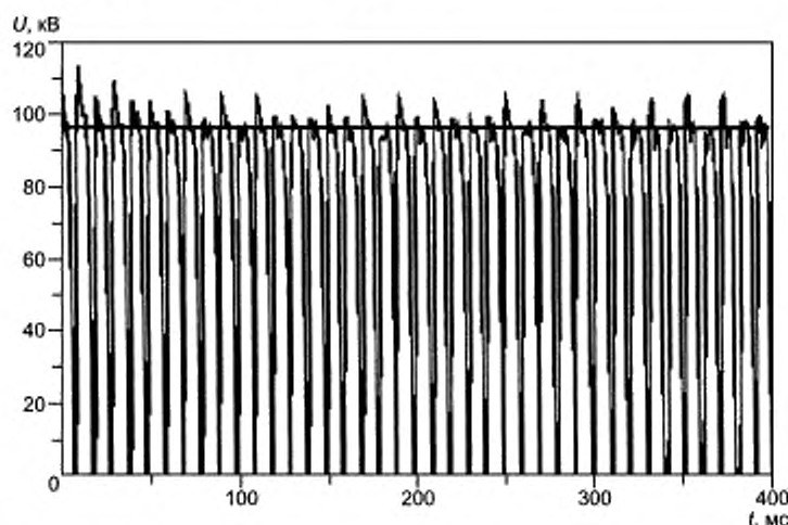
Рисунок В.1 — Пример выходного напряжения для двухимпульсного генератора
