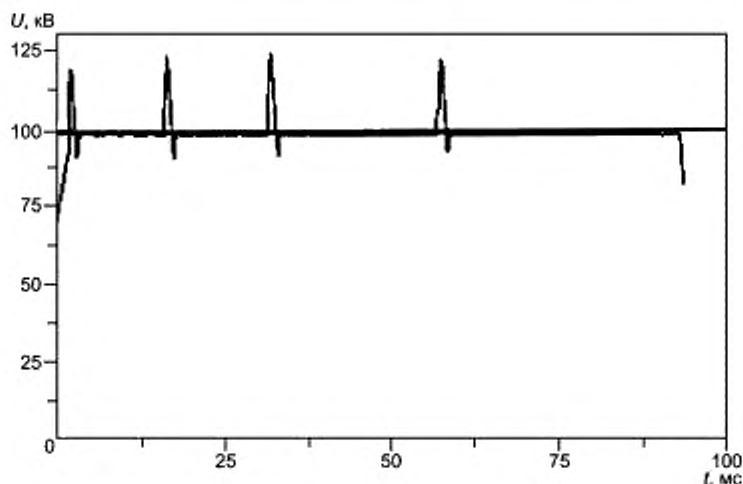
Рисунок В.2 — Пример выходного напряжения для генератора с выходным постоянным напряжением
