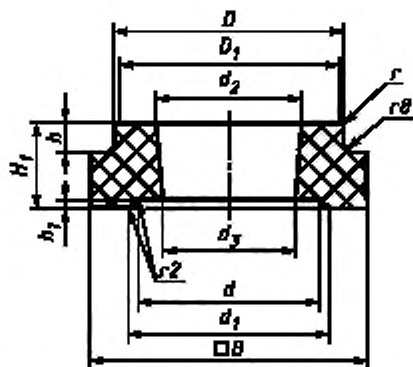
Рисунок 27 — Гнездовой кирпич номер 13 (нижняя часть)
