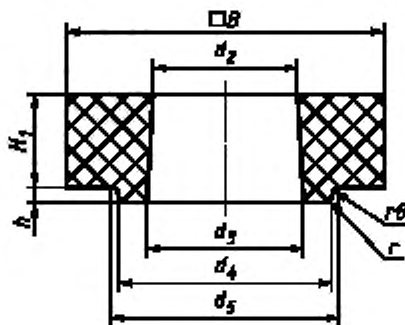
Рисунок 18 — Гнездовой кирпич номер 2 (нижняя часть)
