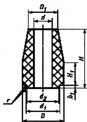
Рисунок 9 — Стакан и стакан-коллектор номеров 9-1 и 9-2
