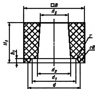
Рисунок 22 — Гнездовой кирпич номер 8 (верхняя часть)
