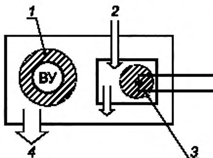
1 — зона, в которой проводится испытание разбавления; 2 — вход продувочного инертного газа; 3 — потенциальный источник утечки с номинальной зоной разбавления; 4 — выход продувочного газа
