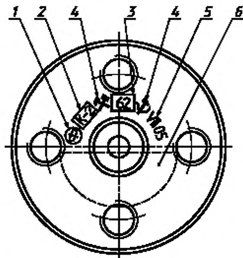
1 — знак формирования; 2 — клеймо ОТК, 3 — условный номер предприятия, сформировавшего колесную пару; 4 — приемочные клейма представителя потребителя; 5 — дата формирования; 6 — клейма, относящиеся к изготовлению оси
