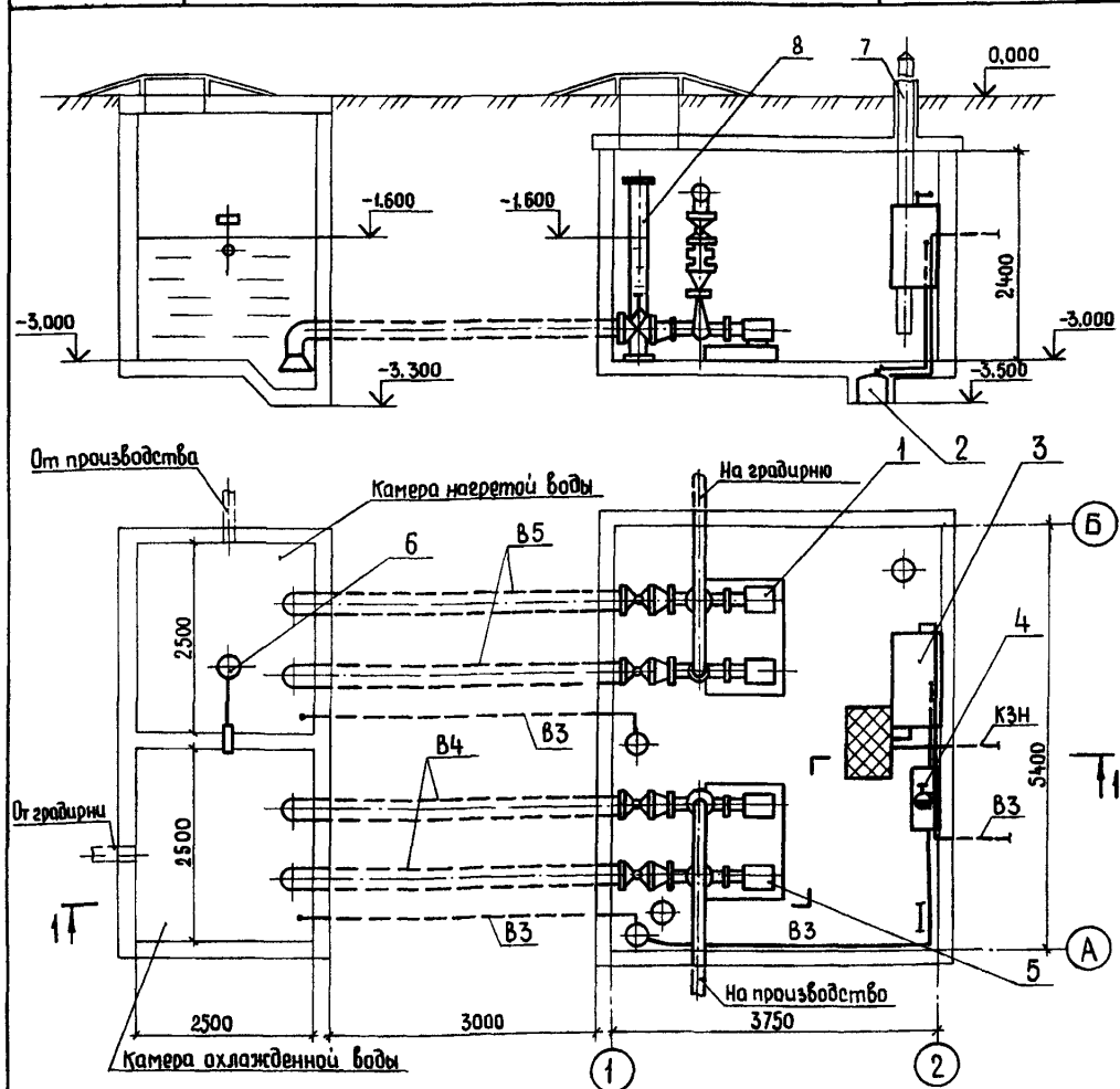
ЭКСПЛИКАЦИЯ ОБОРУДОВАНИЯ
