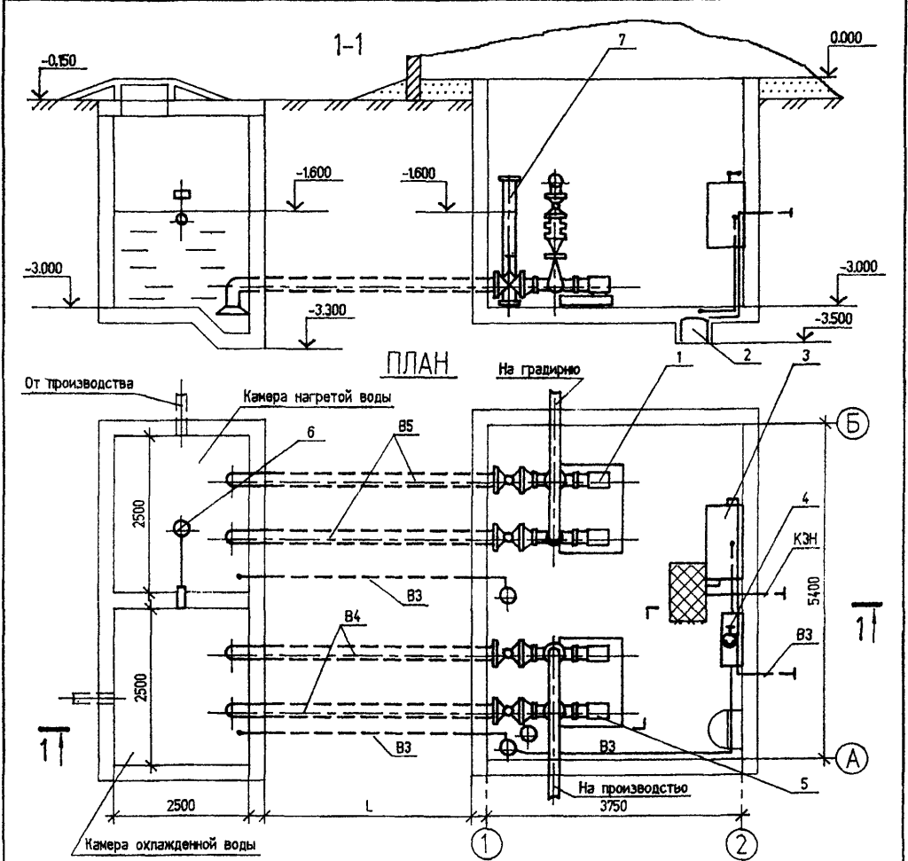
ЭКСПЛИКАЦИЯ ОБОРУДОВАНИЯ
