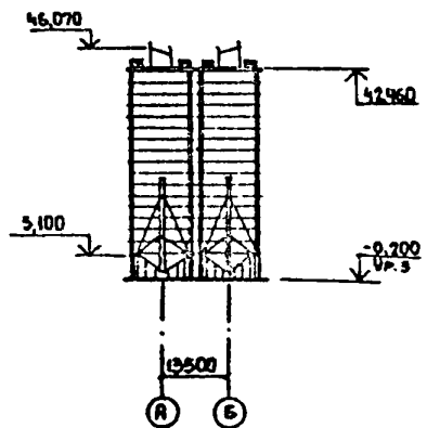
Разрез I-I
