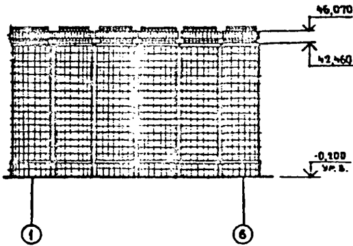
Пример компоновки двухрядного сiloсного корпуса емкостью 32 тыс.т
