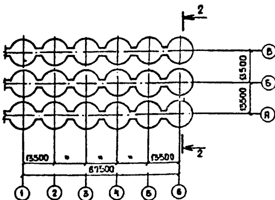
Пример компоновки трехрядного сiloсного корпуса емкостью 48 тыс.т
