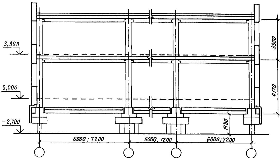
Разрез по зданию с техническим подпольем над холодным подпольем (Здание типа 3г)
