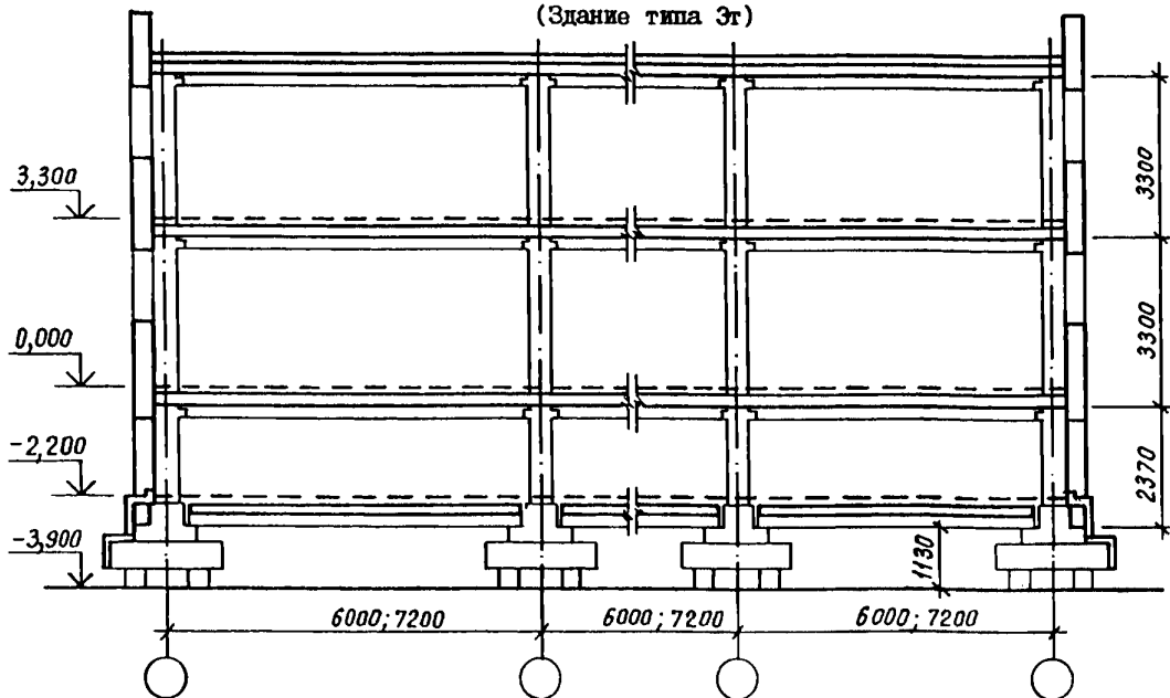
Разрез по зданию с техническим подпольем над холодным подпольем (Здание типа 3г)
