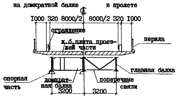
Поперечный разрез
