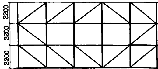
План продольных связей. Г-10(Г-11,5)
