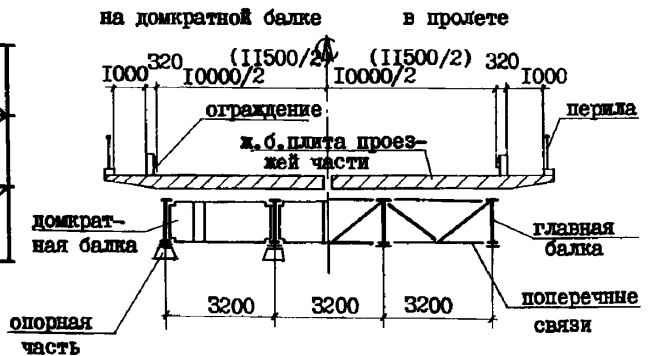
Поперечный разрез
