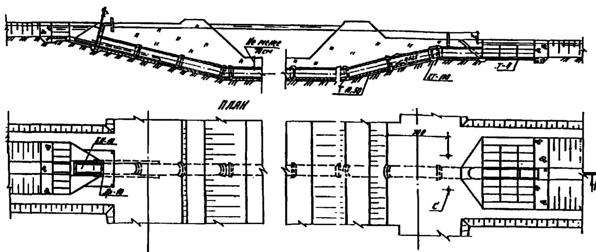
РАЗРЕЗ I-I
