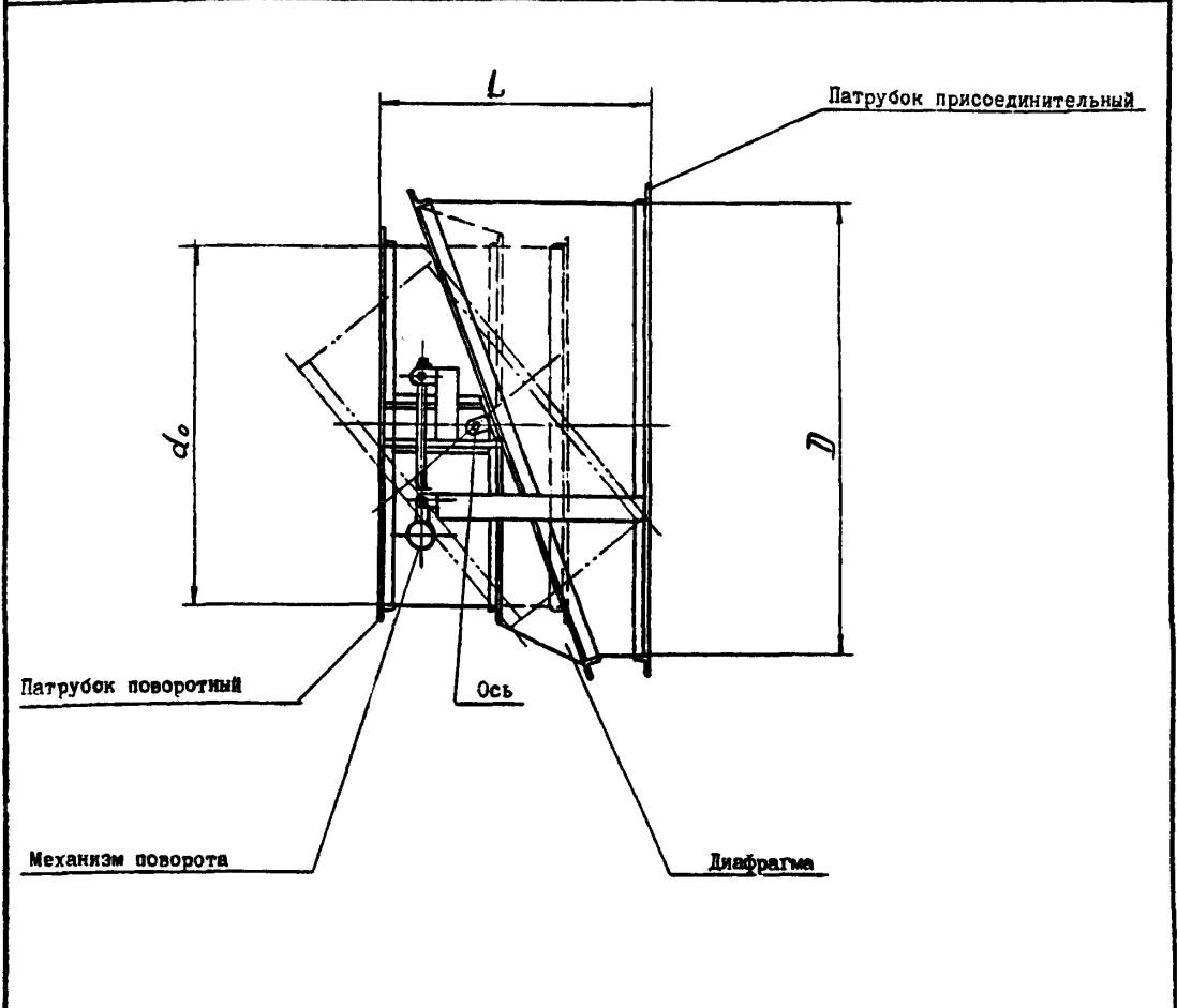
Д 1АА ТЕХНИЧЕСКАЯ ХАРАКТЕРИСТИКА ОСНОВНЫХ ПАРАМЕТРОВ ВОЗДУХОРАСПРЕДЕЛИТЕЛЕЙ
