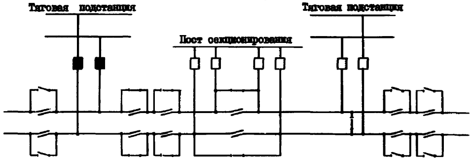
ПРИНЦИПАЛЬНЫЕ СХЕМЫ ДЛЯ ПЛАКИ ГОЛОМЕДА НА КОНТАКТНОЙ СЕТИ
