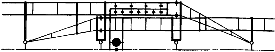
ПРИНЦИПАЛЬНЫЕ СХЕМЫ ДЛЯ ПЛАКИ ГОЛОМЕДА НА КОНТАКТНОЙ СЕТИ
