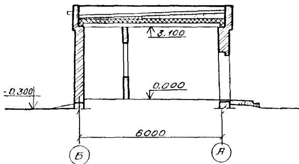
РАЗРЕЗ I - I
