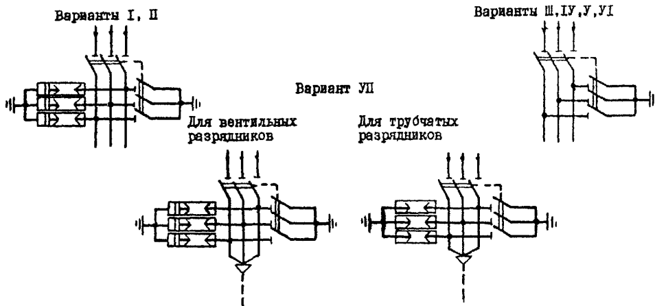
Схемы электрических соединений РП
