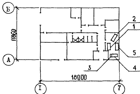
ПЛАН РАЗМЕЩЕНИЯ ТЕХНОЛОГИЧЕСКОГО ОБОРУДОВАНИЯ
