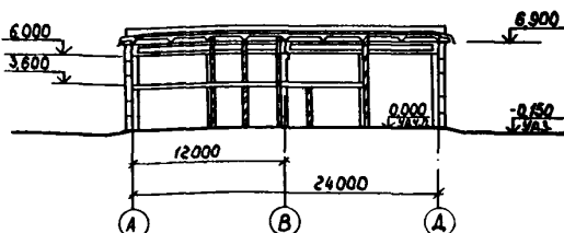
Р А З Р Е З 2-2
