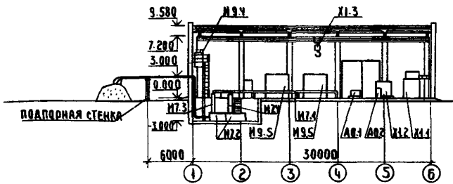
РАЗРЕЗ I-I
