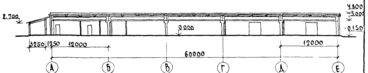
РАЗРЕЗ I-I
