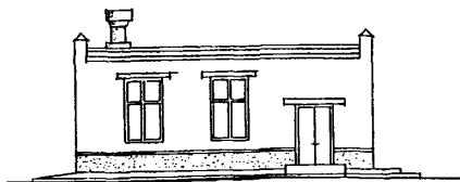
ФАСАД I-2
