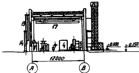
РАЗРЕЗ I-I
