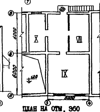
ПЛАН НА ОТМ. +0,360
