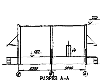
РАЗРЕЗ А-А
