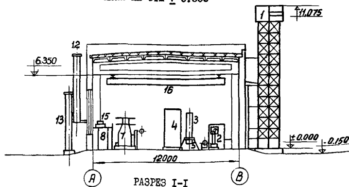
РАЗРЕЗ I-I
