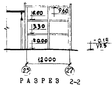
РАЗРЕЗ 2-2
