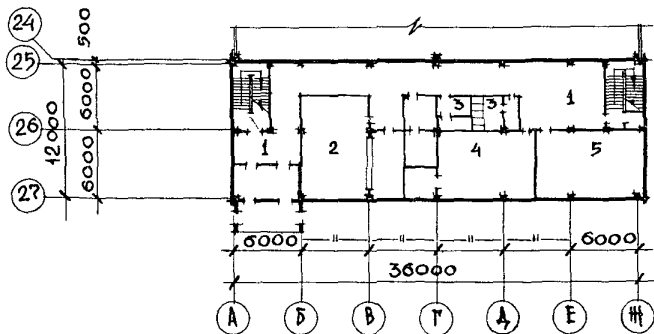
План на 000
