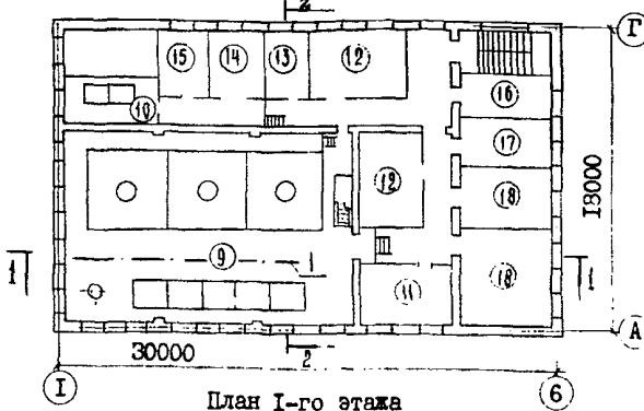
План I-го этажа
