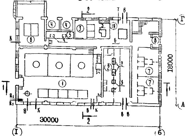
План I-го этажа
