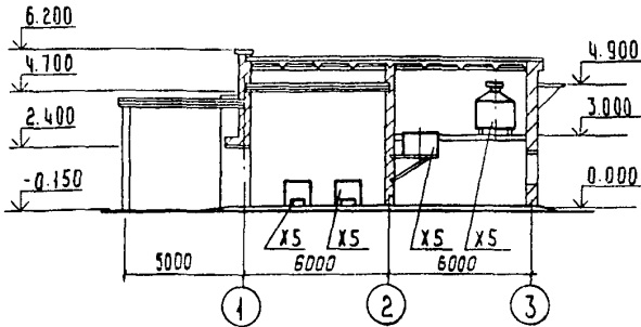
РАЗРЕЗ I-I
