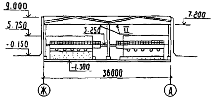
РАЗРЕЗ 2-2
