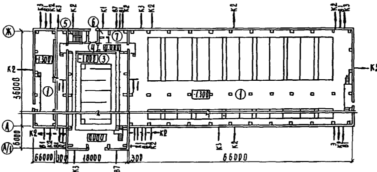
ПЛАН НА ОТМ.-1.300 И 0.000
