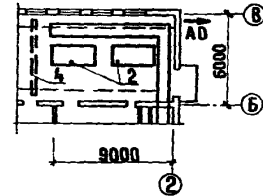
ЭЛЕМЕНТ ПЛАНА НА ОТМ. 0,000 (ВАРИАНТ С ТУРБОВОЗДУХОВКАМИ)
