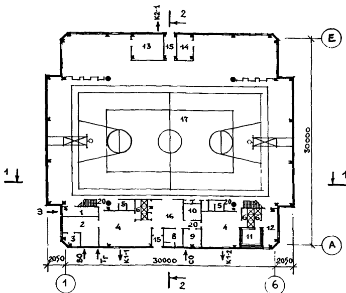
ЭКСПЛИКАЦИЯ ПОМЕЩЕНИЙ
