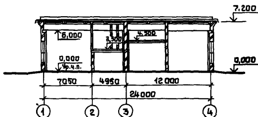
Р А З Р Е З I-I
