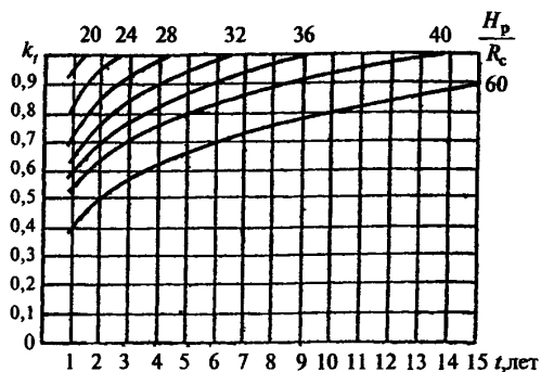
Рис. 2. Графики для определения коэффициента k_t при t от 1 года до 15 лет
