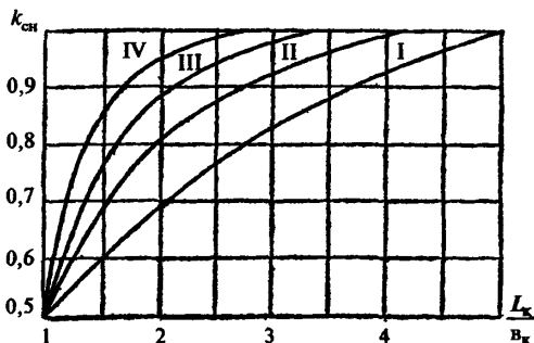
Рис. 6. Графики для определения коэффициента k_{\text{сн}} L_k — длина камеры, B_k — ширина камеры, I, II, III, IV — категории устойчивости пород
