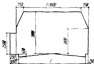
Рис. 1. Габарит приближения конструкций автодорожных тоннелей
