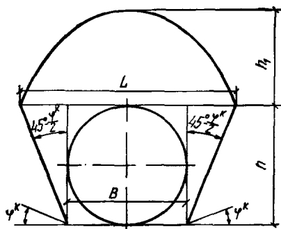
Рис. 2. Схема свода обрушения
