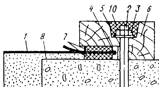
Рис. 6. Сопряжение пленочного элемента с бетонными сооружениями
