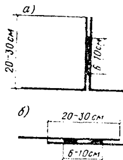
Рис. 8. Двойные сварные швы
