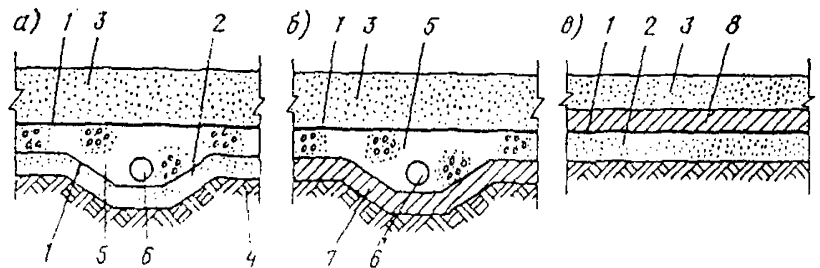
Рис. 3. Конструкции двухслойного (а, б) и комбинированного (в) противофильтрационного устройства из полиэтиленовой пленки
