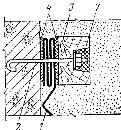
Рис. 7. Конструкции устройства для закрепления пленочного (листового) элемента
