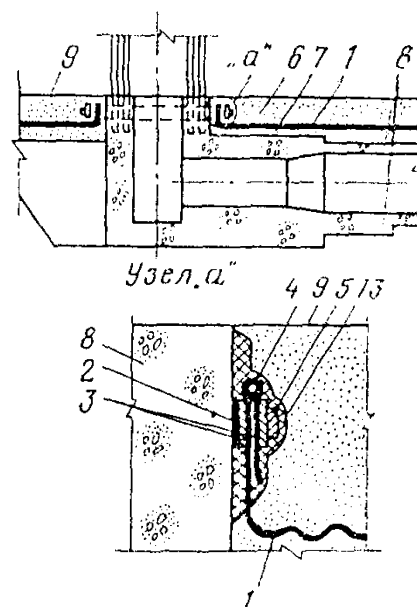
Рис. 4. Сопряжение пленочного элемента с бетонным водосбросным колодцем
