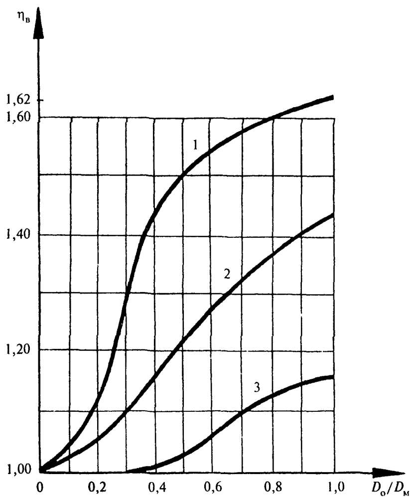
ГРАФИК ДЛЯ ОПРЕДЕЛЕНИЯ КОЭФФИЦИЕНТА НЕСУЩЕЙ СПОСОБНОСТИ ТРОЙНИКОВ \eta_b
